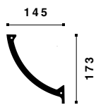
L3 ARSTYL® 173 x 145 x 2000 mm
