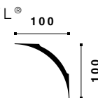
NE4 PURE NOMASTYL® 100 x 100 x 2000 mm
