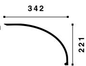
MC1 ARSTYL® 221 x 342 x 2000 mm
