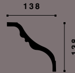
TI NOMASTYL® 138 x 138 x 2000 mm
